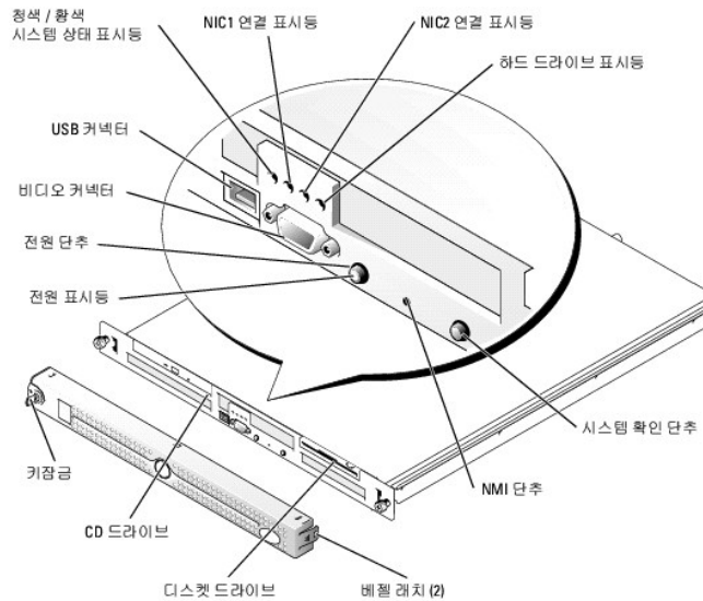
그림 1-1. 전면 패널 구조
